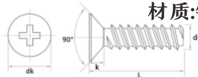
d:代表螺纹直径 L:代表总长度(含头部) k:代表头部厚度 dk:代表头部直径
