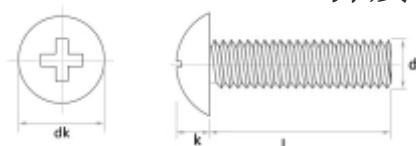
d:代表螺纹直径 L:代表总长度(含头部) k:代表头部厚度 dk:代表头部直径
