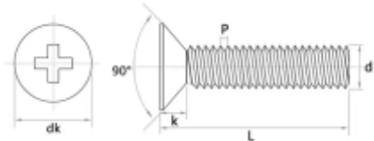
d:代表螺纹 L:代表总长度 p:代表螺距 t:代表内六角深度 s:六角对边距离
