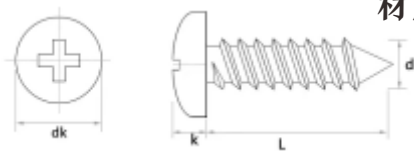
d:代表螺纹直径 L:代表总长度(含头部) k:代表头部厚度 dk:代表头部直径
