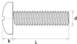
d:代表螺纹直径 L:代表总长度(含头部) k:代表头部厚度 dk:代表头部直径
